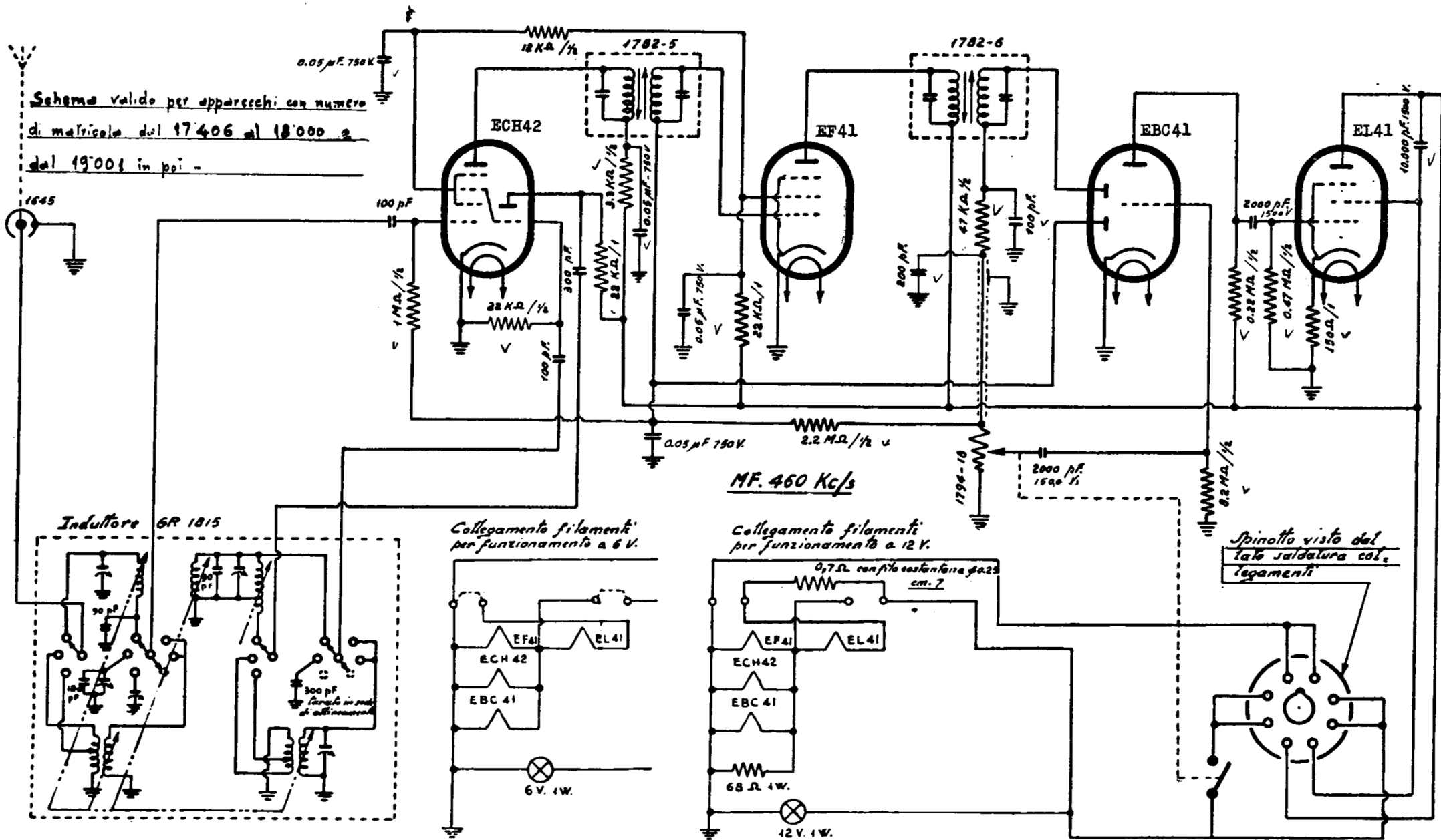
GALLO-CONDOR - Apparecchio autoradio mod. Ultra-plat 3 a serie. Lo schema vale per apparecchi dal n. 17406 al 18000 e dal 19001 in poi. Media frequenza 460 kc,
